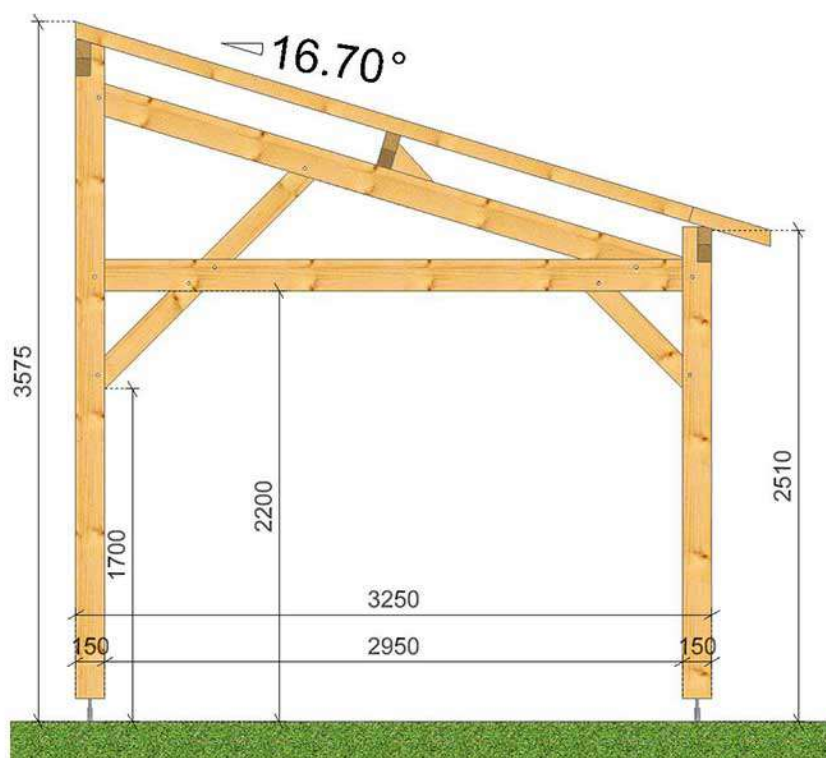
Plan de coupe
