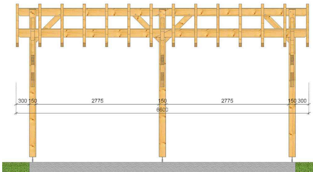
Vue de plan
