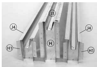
Nur Gr. 5 u. 7 / Sizes 5 and 7 only Taille 5 + 7 / Misura 5 + 7 Dachträger (J4) und Firststütze (H1) Roof beams (J4) and ridge supports (H1) porte-toit (J4) et support de faîtière (H1) trave tetto (J4) sostegno colmo (H1)
