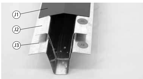
Firstabdeckung (J1) Firstträger oben (J2) Firstträger unten (J3) roof ridge cover (J1) upper roof ridge beam (J2) lower roof ridge beam (J3) couverture de faîtière (J1) poutre de faîtière sup. (J2) poutre de faîtière inf. (J3) copertura colmo (J1) supporto colmo superiore (J2) supporto colmo inferiore (J3)
